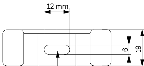
ovales Loch für Schraube zum Befestigen der Halterung
